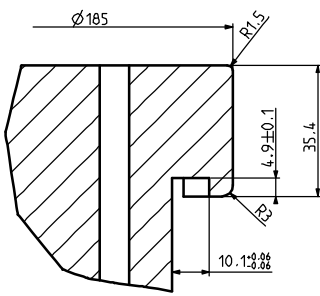
SEZIONE K-K
